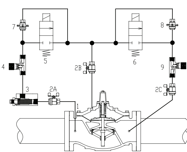
Schematic A-7637A
