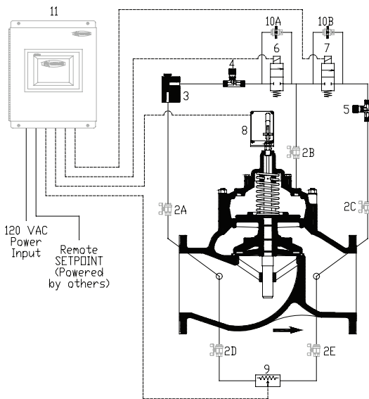
Schematic A-8450C
